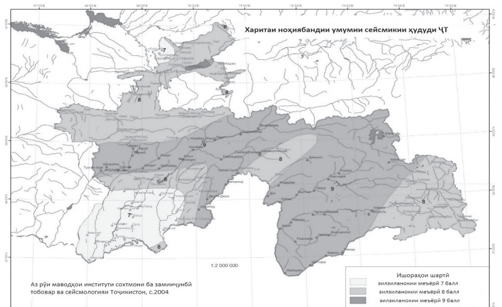
ХАРИТАИ НОҶИЯБАНДИИ УМУМИИ СЕЙСМИКӢ ҲУДУДИ ҶУМҲУРИИ ТОҶИКИСТОН
