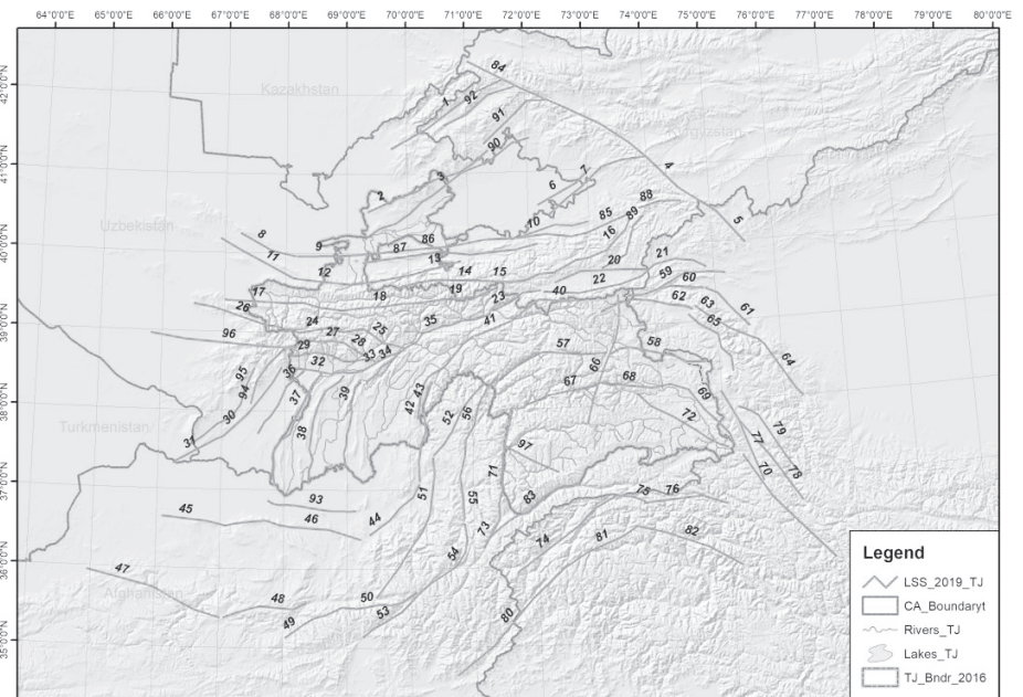
ХАРИТАИ ҶОЙГИРШАВИИ АСОСИ ТАРҚИШҶОИ ЗАМИНИИ ҲУДУДИ ТОҶИКИСТОН ВА ҲАМСАРҶАДИ ОН
